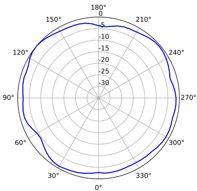
2.4GHz (水平)
