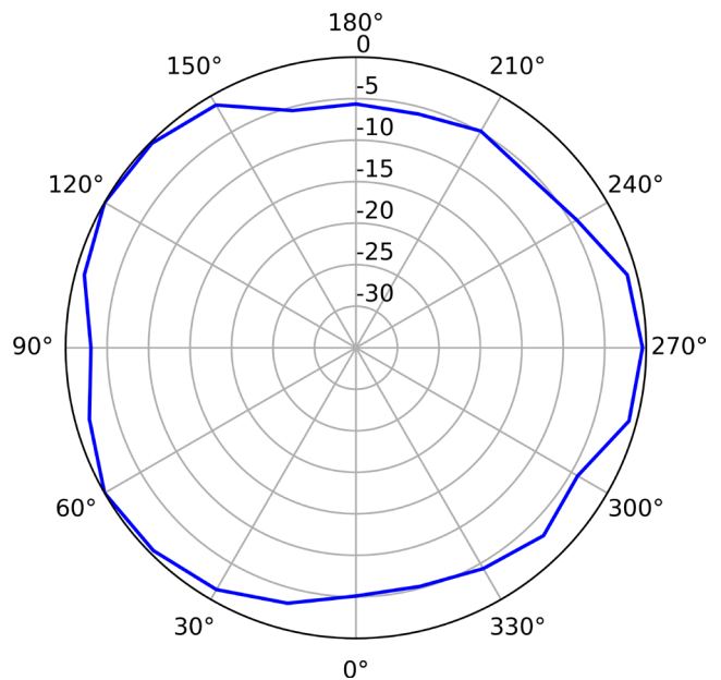
2.4GHz (垂直)
